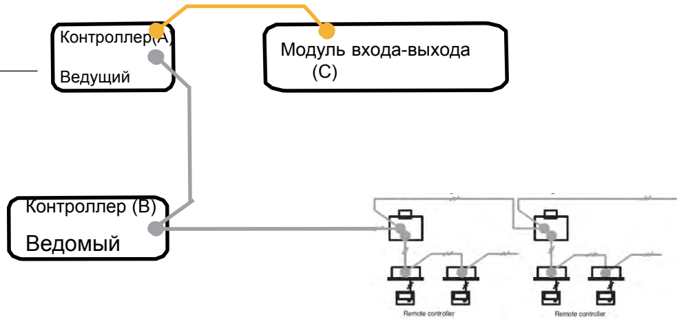
Интегратор
