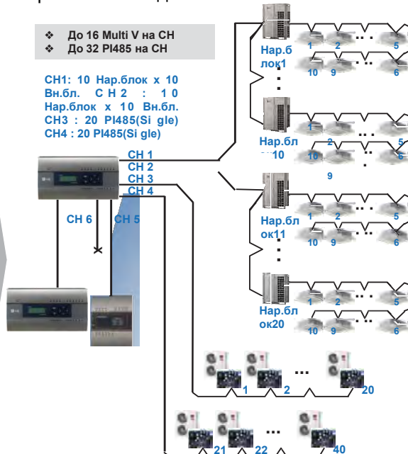
Правильное подключение кабеля
